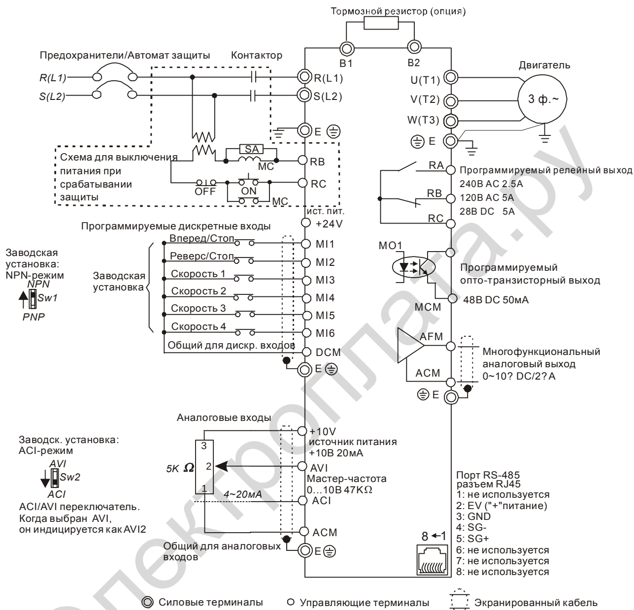
Рисунок 5. Схема для моделей VFD002E11T/21T, VFD004E11A/21T, VFD007E21T.
