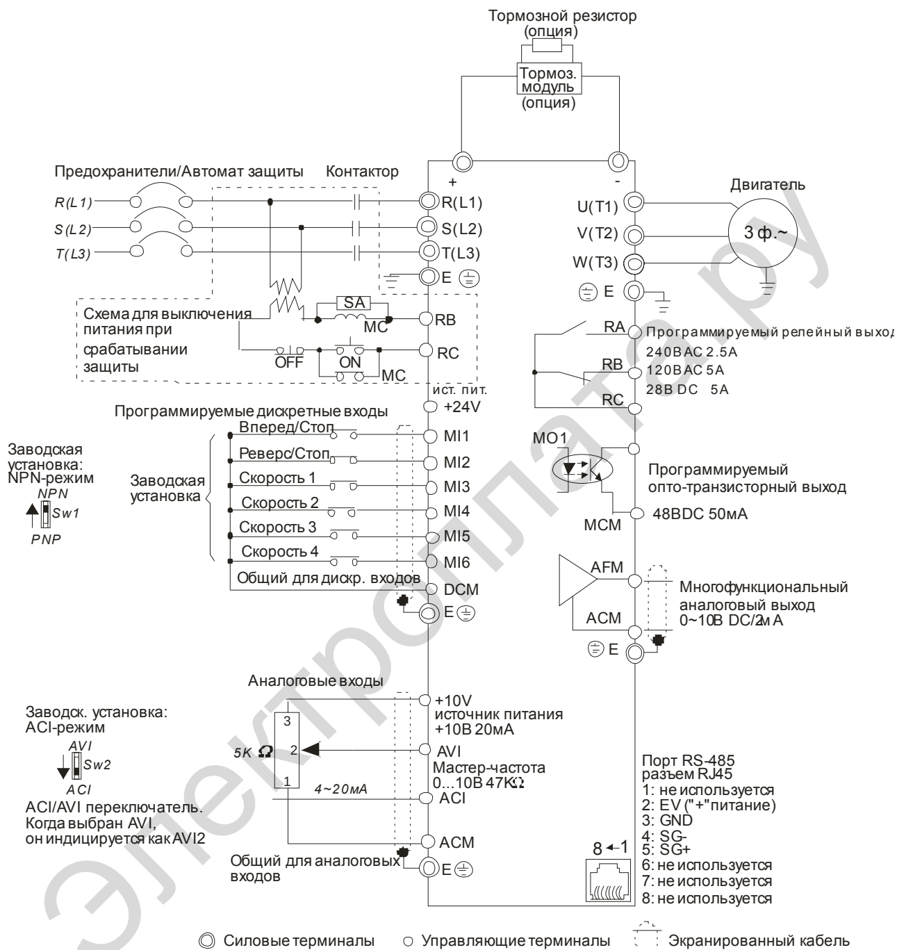
Рисунок 2. Схема для моделей VFD002E23A, VFD004E23A/43A, VFD007E23A/43A, VFD015E23A/43A, VFD002E23C, VFD004E23C/43C, VFD007E23C/43C, VFD015E23C/43C, VFD002E23P, VFD004E23P/43P VFD007E23P/43P, VFD015E23P
